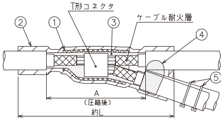
※図面は1相分のみを表示です
